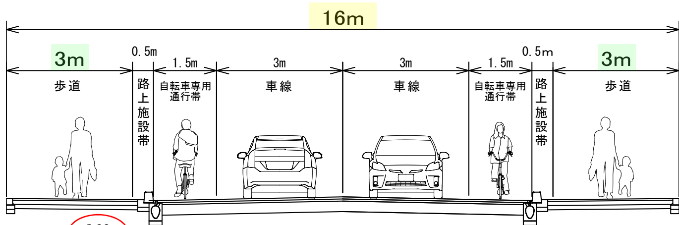
電線共同溝
